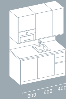
Typ 160
